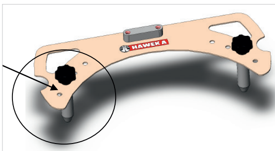
Durch die verstellbaren Aufnahmedorne an der Wasserwaage ist diese nahezu an allen Pkw und L-LKW einsetzbar.
